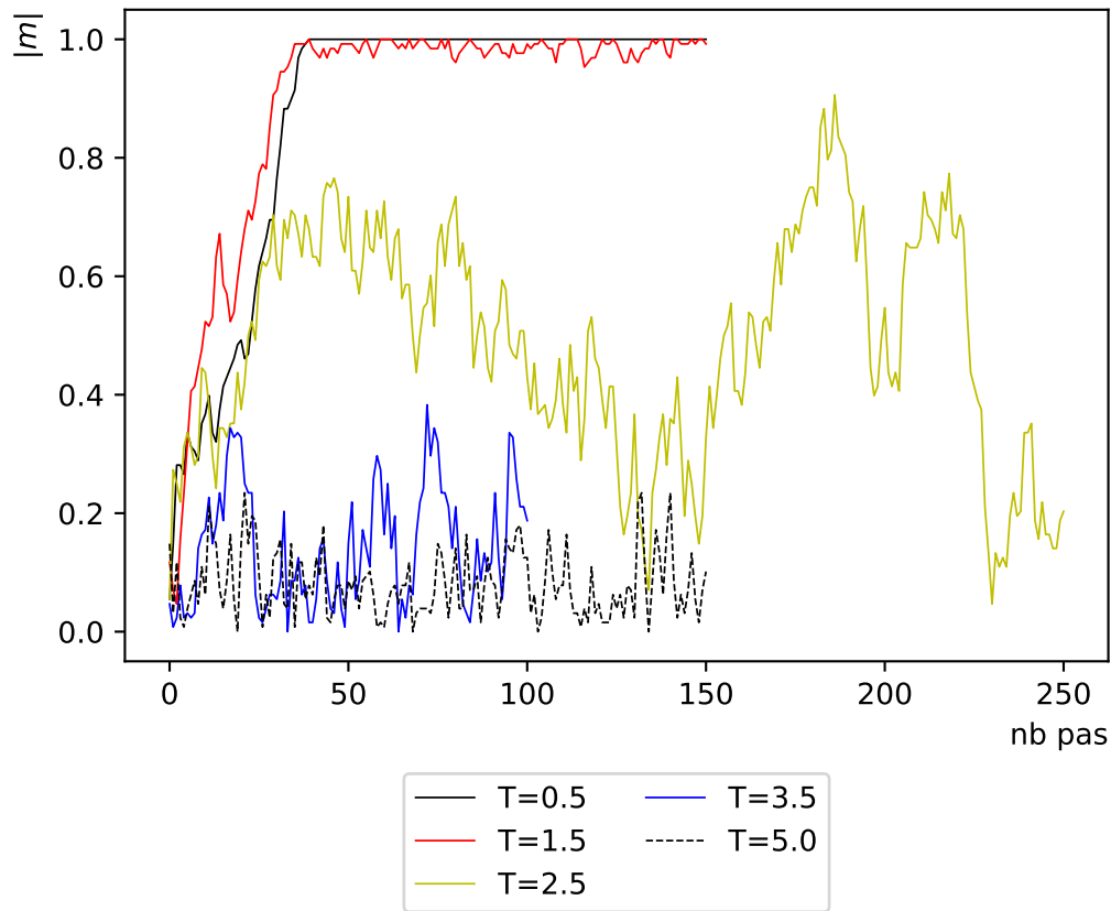
Evolution de l'aimantation sur critère Estimation par intervalle, N=16
